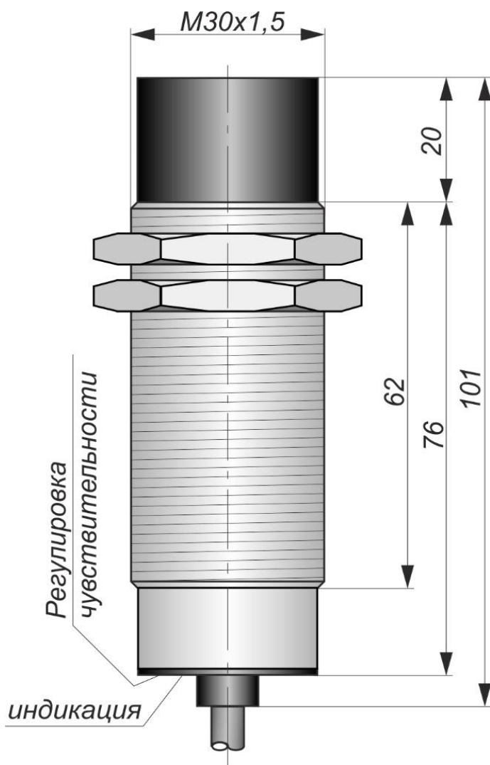
Габаритный чертеж
