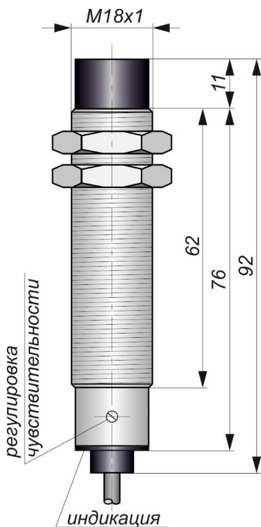
Габаритный чертеж
