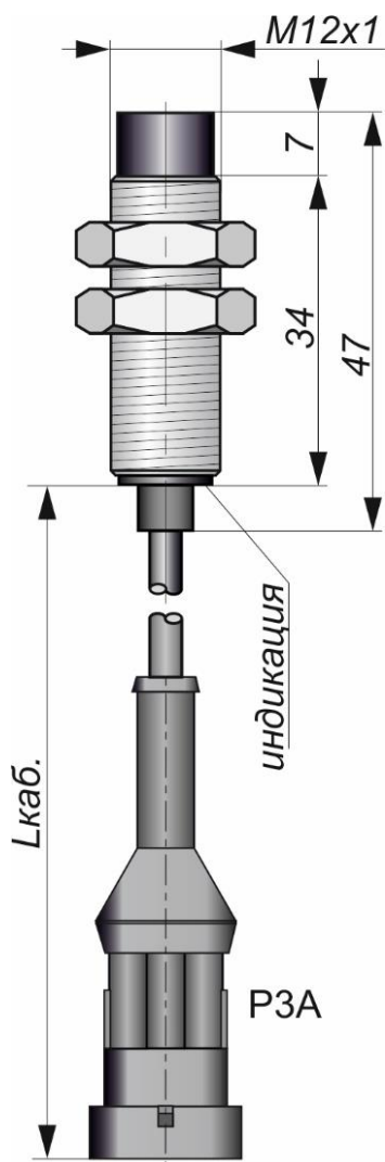
Габаритный чертеж
