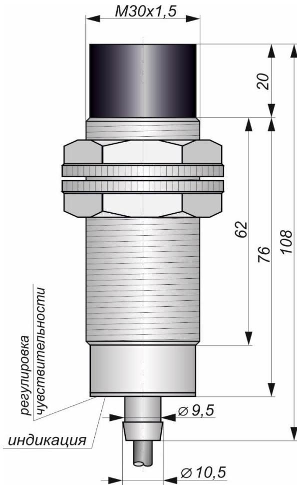
Габаритный чертеж
