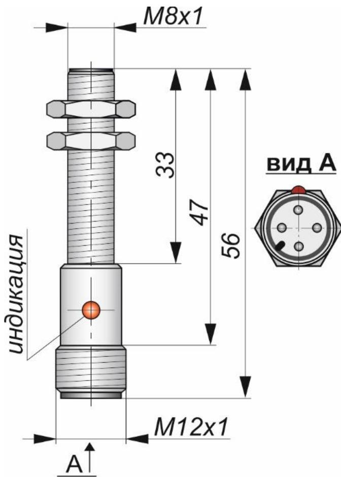
Габаритный чертеж
